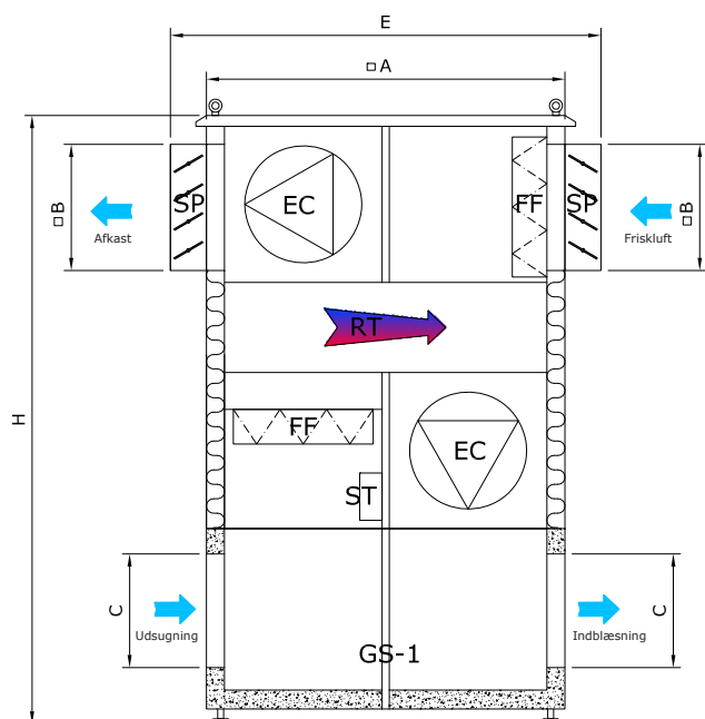
Indendørsmodel med spjæld (Kan laves til udendørsmodel med vejr-skjold på sjældmotorer)
